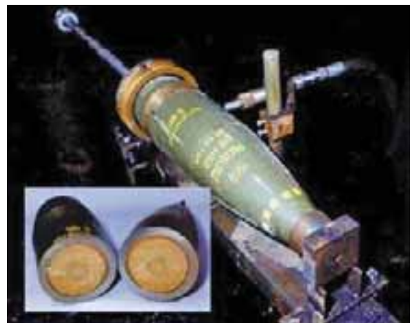
Figure 5.3 : Équipement pour le découpage hydro-abrasif, et coupe d'un obus de 155 mm
