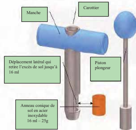
Figure 3: Exemple d'un kit de carottage de sol
