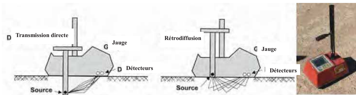
Figure 4: Présentation du principe de fonctionnement du densimètre nucléaire [7] et le densimètre nucléaire PortaProbe CPN MC-3, utilisé par le Centre suédois SWEDEC
