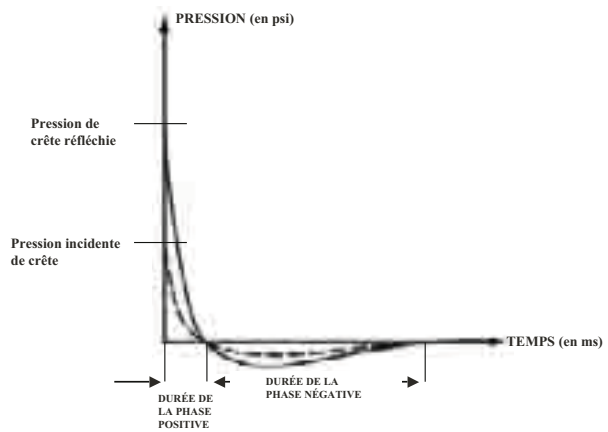
Courbe Pression-Temps
